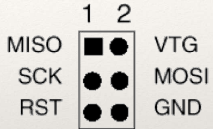
Conector ICSP (linha Arduíno)
