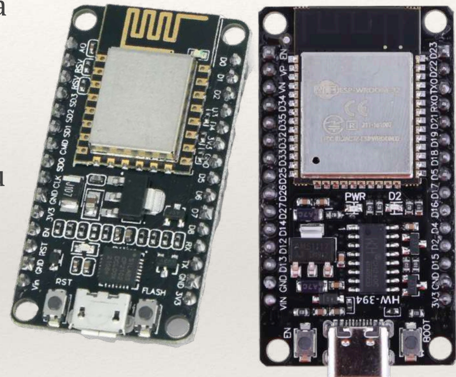
ESP8266 Node MCU e ESP32 WROOM, duas das placas de protótipo mais populares da Espressif
