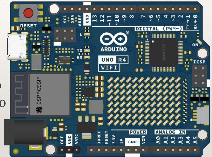
Arduíno Uno R4 Wi-Fi
