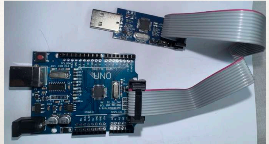
Programador USBasp em um Arduíno Uno
