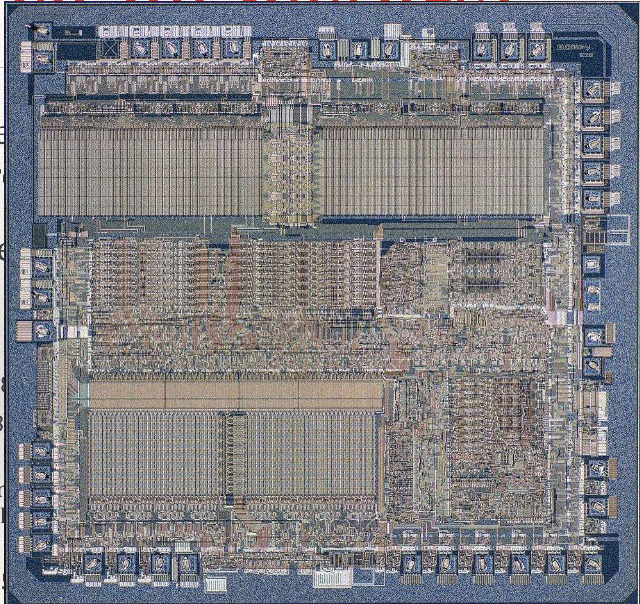
Microcontrolador Intel 8051
